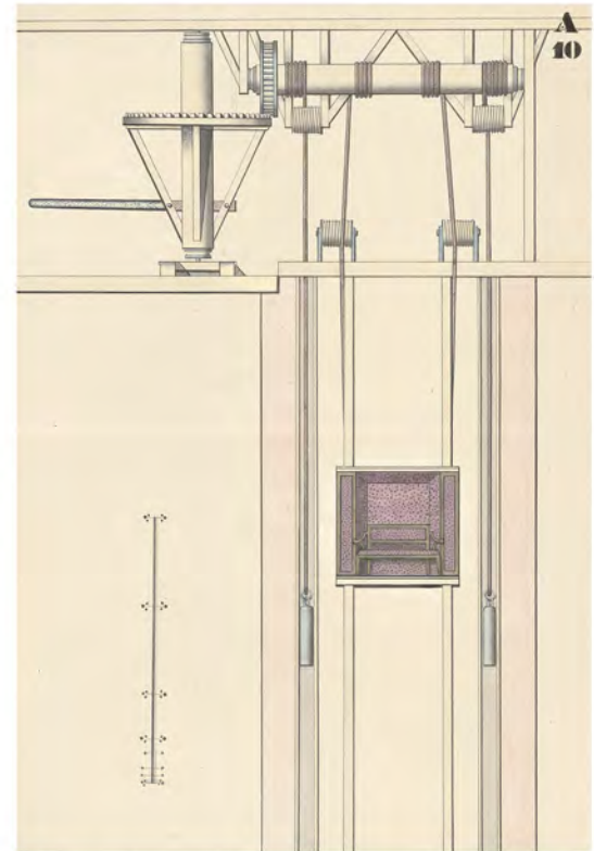
232 | Aufzugmaschine mit Liftkabine, um 1773. Kolorierte Federzeichnung/Gouache auf Papier (Albertina Wien, Inv.Nr. AZ 9601)
